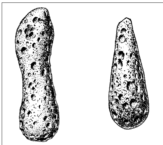
Indonesian tektites
